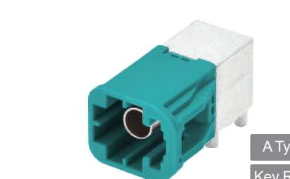
542 Mini FAKRA Plug 1x1 Right Angle Type Coding:A,B,C,D,E,F,G,H,J,K,N,Z Positions:01
