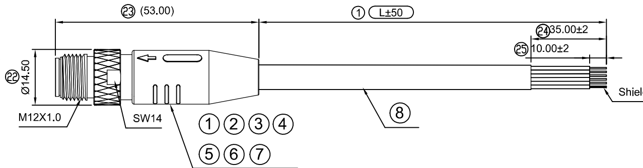
A-Code(5pin)
