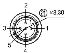
A-Code(5pin)
