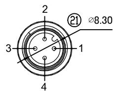
A-Code(4pin)
