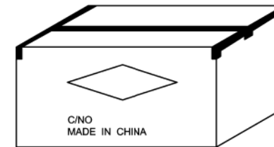
(CARTON:L457*W298*H228mm,Material K=K) (200PCS CABLE/CARTON)
