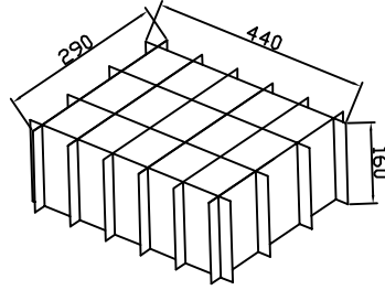
(刀卡組裝圖)
