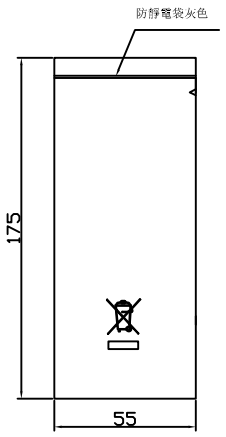
( 防靜電袋 )
