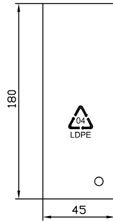
PE BAG:L180mmx45mmxT0.03mm.
