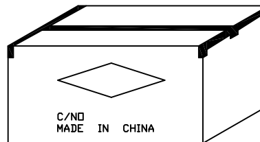
(CARTON:L457*W298*H228mm,Material K=K)
