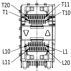
DETAIL A 1:1
