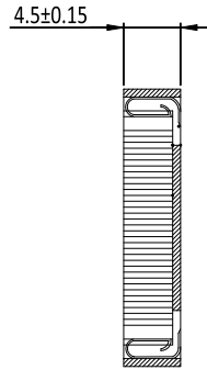
SECTION A-A
