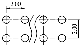
P.C.B. LAYOUT
