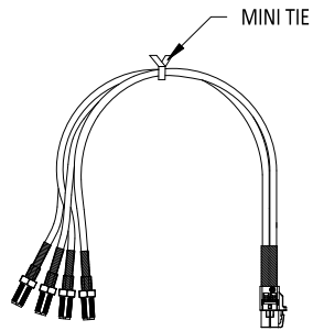
MINI FAKRA A 2x2 JACK TO SMA JACK x4 CABLE
