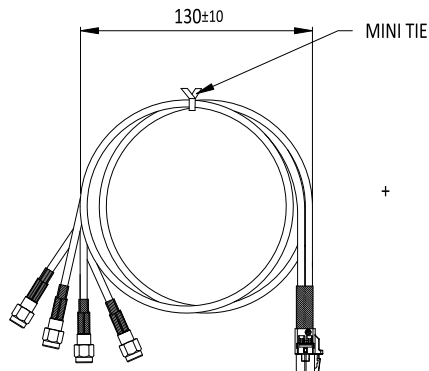
MINI FAKRA A 2x2 JACK TO SMA PLUG x4 CABLE
