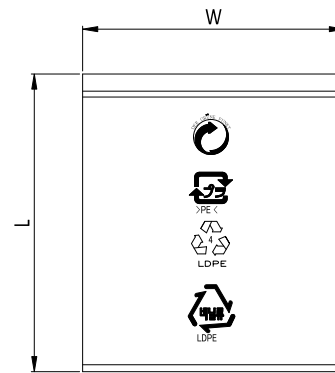
ZIP BAG: L203xW165xT0.05mm
