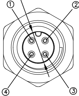
A-Code(4pin)
