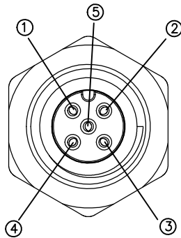
A-Code(5pin)
