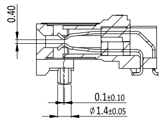
剖面圖 A-A
