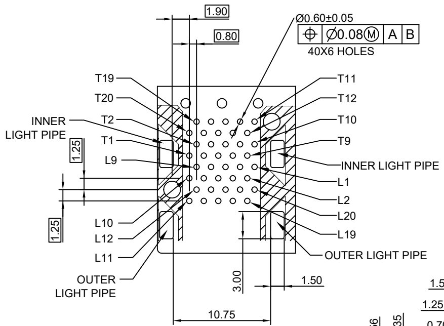
DETAIL H 2:1
