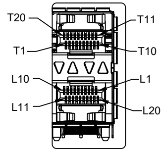
DETAIL A 1:1
