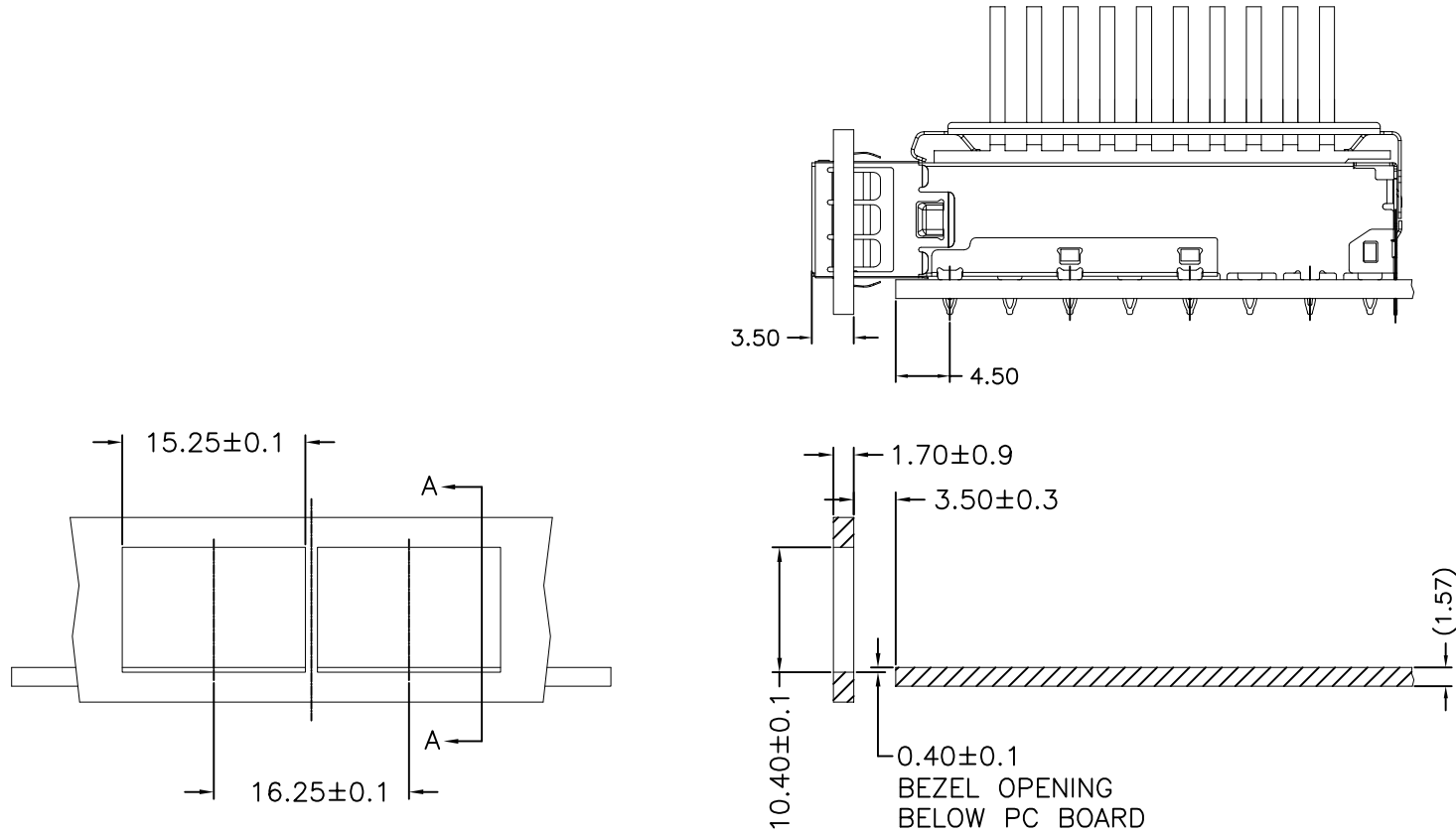
SECTION A-A
