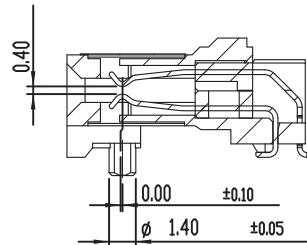
剖面圖 A-A
