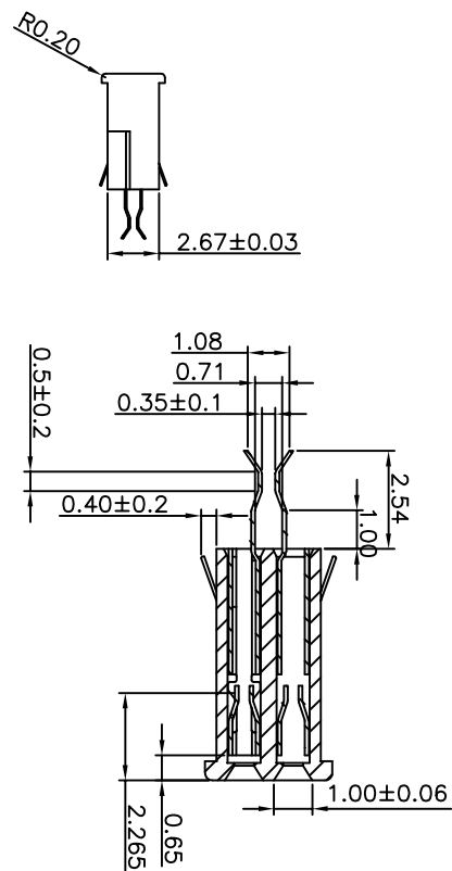
A-A(SCALE 2:1)
