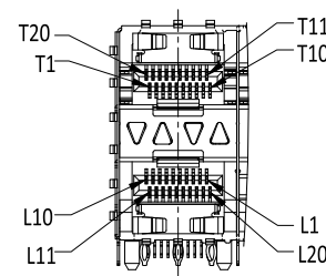
DETAIL A 1:1
