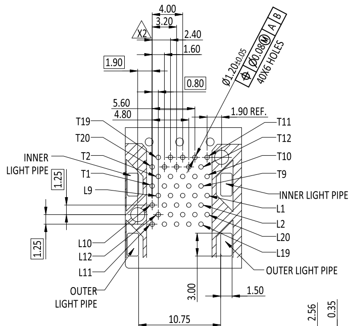
DETAIL H 2:1
