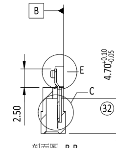
剖面圖 B-B
