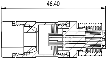
剖面圖 A-A
