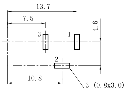
PCB板安裝尺寸示意圖
