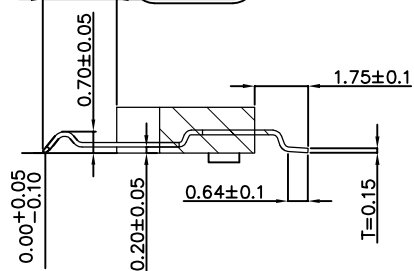
A-A SECTION
