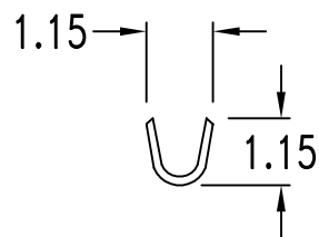
SEC. A-A
