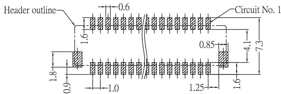
P.C.B. LAYOUT
