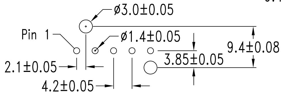
P.C.B. hole dimensions
