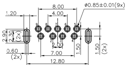
P.C.B LAYOUT TOL: 1.20 ± 0.05
