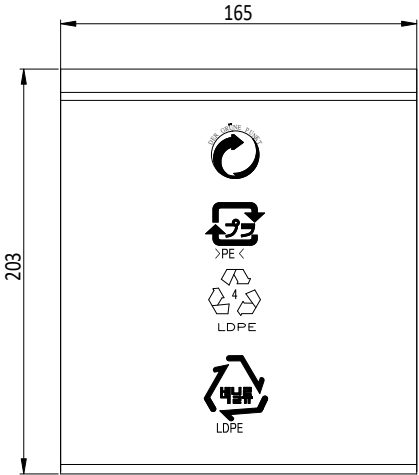
ZIP BAG: L203xW165xT0.05mm
