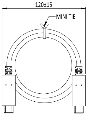
USB C/C 3.1 CABLE
